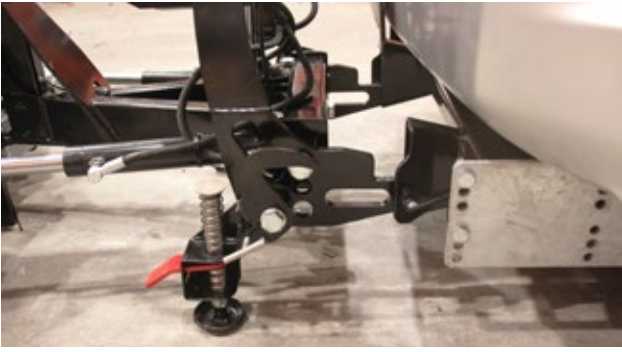
Quick hitch - lyft handtaget för att haka fast plogen till bilen
